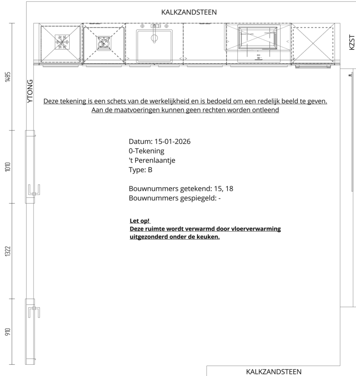
WANDAANZICHT A
